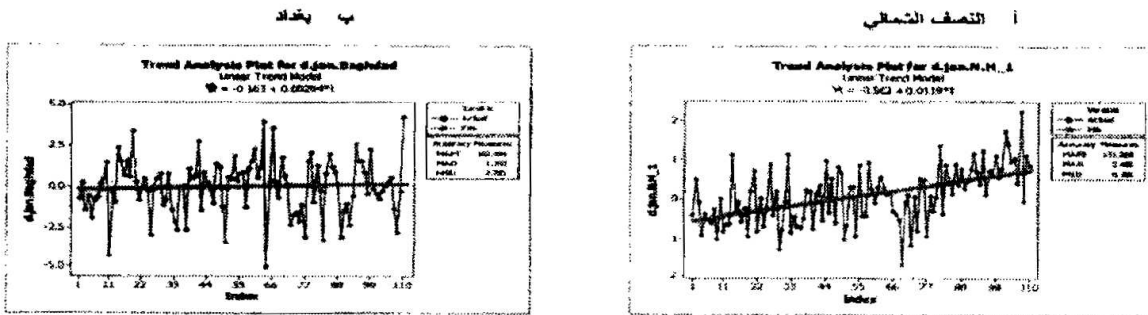
شكل رقم (٦) انحرافات المعدل السنوي العام لدرجات الحرارة ١٩٠١-٢٠١٠
