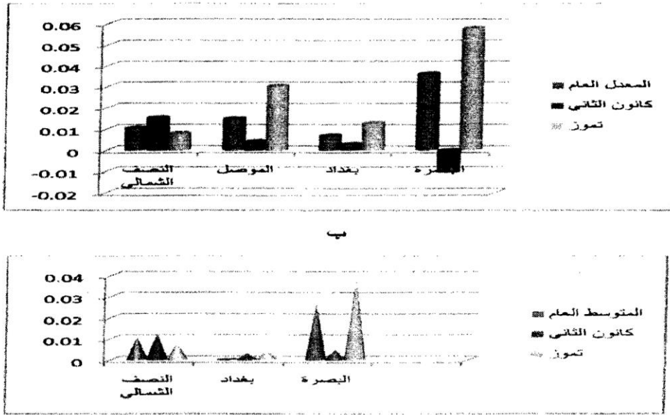
شكل رقم (٩) انحرافات معدلات درجات الحرارة
