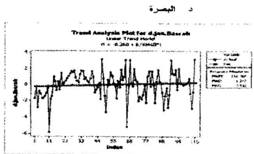
شكل رقم (٧) انحرافات معدلات شهر كانون الثاني ١٩٠١-٢٠١٠
