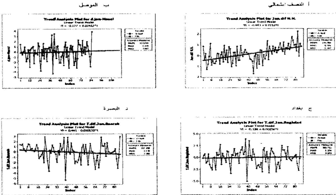
شكل رقم (٣) انحرافات معدلات درجات الحرارة لشهر كانون الثاني ١٩٢٦-٢٠١٠
