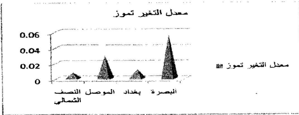
شكل رقم (٥) انحرافات معدلات درجات الحرارة للمدة ١٩٢٦-٢٠١٠
