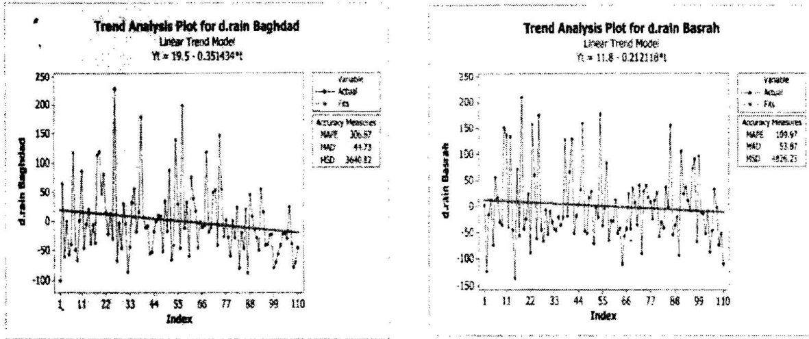
شكل رقم (١٢) انحرافات معدلات كميات الامطار لمخطي بغداد والبصرة للمدة ١٩٠١-٢٠١٠
